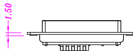
Receptacle Contact
