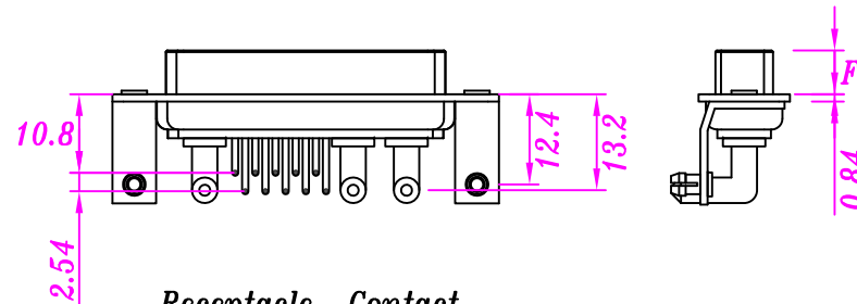
Receptacle Contact
