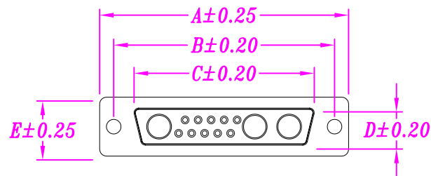
Receptacle Contact
