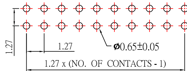
P.C.Board Layout
