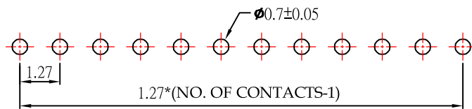
P.C.Board Layout
