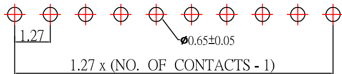
P.C.Board Layout
