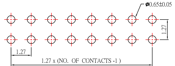
P.C.Board Layout
